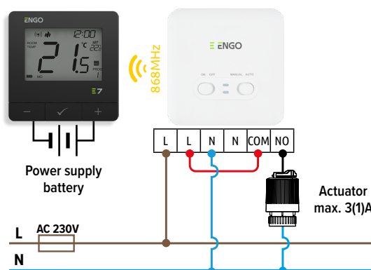
c) Diagrama de conexiune pentru actuator
