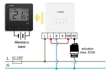
c) Diagrama de conexiune pentru actuator
