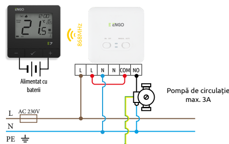
b) Diagrama de conexiune pentru pompele de circulație
