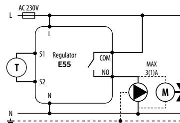
c) Schemat podłączenia do listwy sterującej
