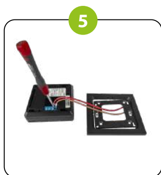
5 Podłącz przewody do regulatora
