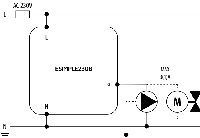
a) Schemat podłączenia do pompy / siłownika
