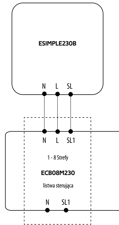
b) Schematy podłączenia do listwy sterującej
