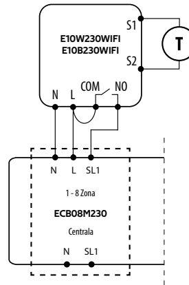
c) Šema povezivanja sa centralom
