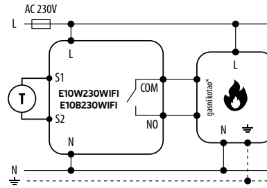
a) Šema povezivanja termostata sa gasnim kotlom
