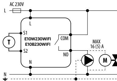
b) Šema povezivanja sa pumpom / aktuatom
