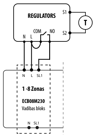
c) Vadības bloka savienojuma shēma
