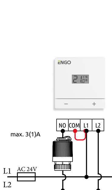
b) Schemat podłączenia do siłownika 24V
