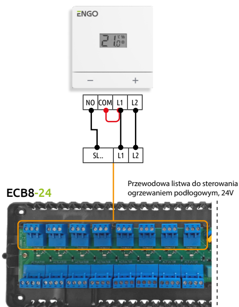
c) Podłączenie urządzeń do listwy sterującej ogrzewaniem podłogowym
