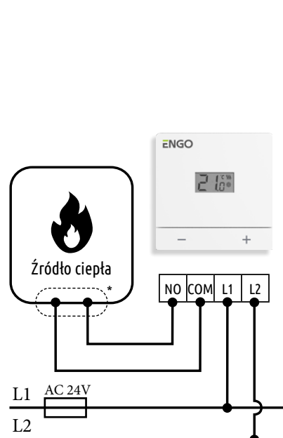
a) Schemat podłączenia do źródła ciepła
