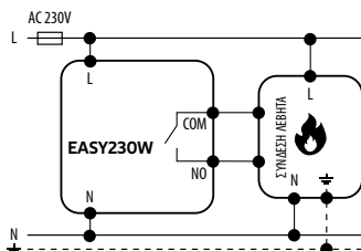
α) Διάγραμμα σύνδεσης στο λέβητα αερίου
