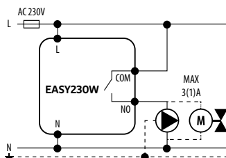
β) Διάγραμμα σύνδεσης σε αντλία / ενεργοποιητή
