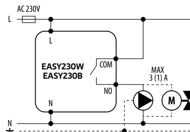
b) Sūkņa/piedziņas elektroinstalācijas shēma
