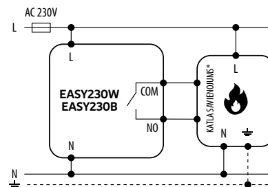
a) Gāzes katla savienojuma shēma
