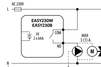
b) Sūkņa/piedziņas elektroinstalācijas shēma
