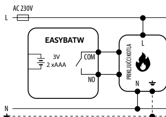
c) Šema povezivanja sa centralom
