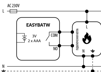
а) Схема підключення до котла
