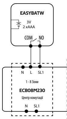
в) Схема підключення до центру комутації
