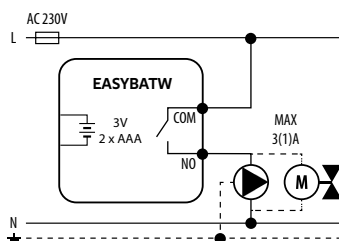
б) Схема підключення до котла
