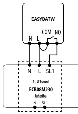
c) Ühendusskeem juhtribale
