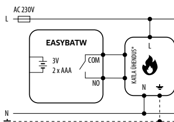
a) Ühendusskeem gaasikatlale
