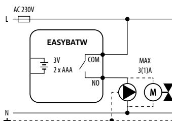
b) Ühendusskeem pumbale / ajamile
