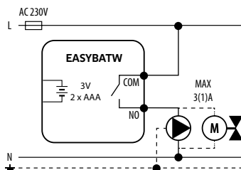
b) Shema priključka na pumpu / aktuator
