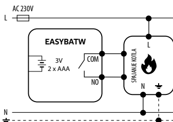
a) Shema priključka na plinski kotao
