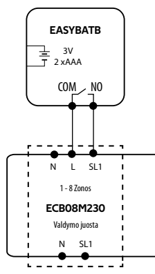
c) Prijungimo prie valdymo juostos schema
