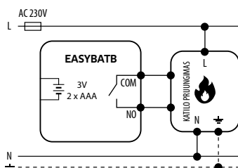
a) Prijungimo prie dujinio katilo schema
