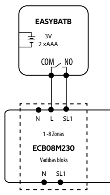
c) Vadības bloka savienojuma shēma
