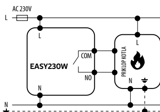
a) Vežalna shema za plinski kote
