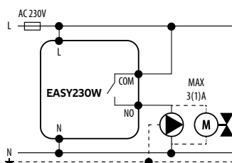
b) Vežalna shema za črpalke/pogon
