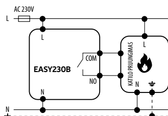
a) Prijungimo prie dujinio katilo schema
