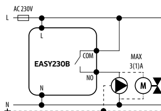
b) Prijungimo prie siurblio / pavaros schema
