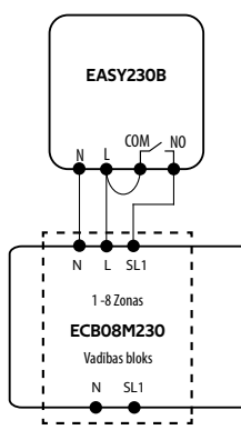
c) Vadības bloka savienojuma shēma
