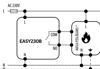
a) Gāzes katla savienojuma shēma
