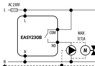
b) Šema povezivanja sa pumpom / aktuatomom
