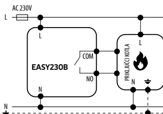
a) Šema povezivanja termostata sa gasnim kotlom
