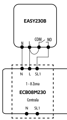
c) Šema povezivanja sa centralom
