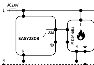
a) Vezalna shema za plinski kote
