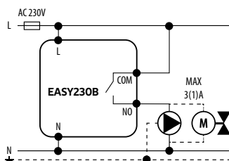
b) Vezalna shema za črpalke/pogon
