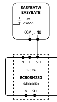
c) schéma zapojenia do ovládacej lišty
