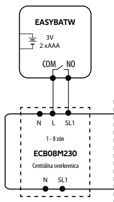
c) Schéma pripojenia k centrálnej svorkovnici
