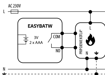
a) Schéma pripojenia k plynovému kotlu
