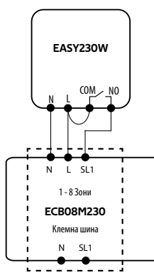
в) Схема на свързване към клемна шина
