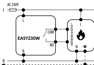
а) Схема на свързване към котел
