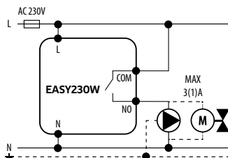
b) Schéma pripojenia k čerpadlu/ovládaču
