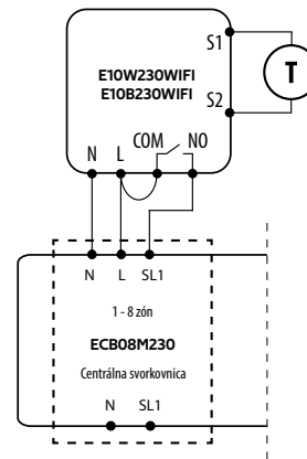
c) Schéma pripojenia k centrálnej svorkovnici
