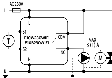
b) Schéma pripojenia k čerpadlu/ovládaču
