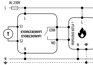
a) Schéma pripojenia k plynovému kotlu
