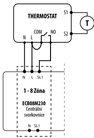
c) Schéma připojení k ústřední svorkovnici
