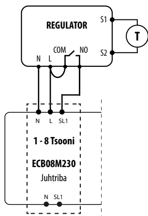
c) Ühendusskeem juhtribale
