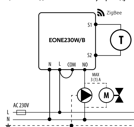
b) Схема подключения к насосу/приводе
