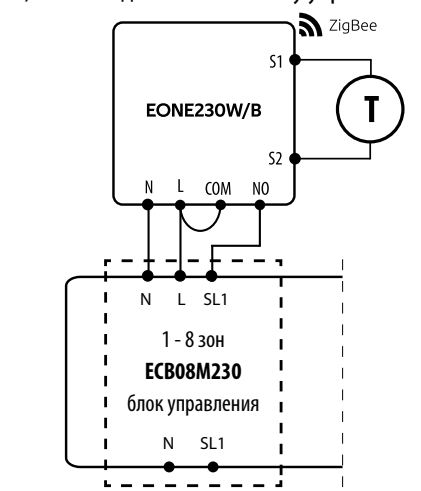
c) Схема подключения к блоку управления
