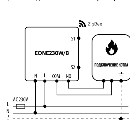
c) Схема подключения к блоку управления
