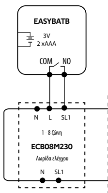
γ) Διάγραμμα σύνδεσης στην λωρίδα ελέγχου
