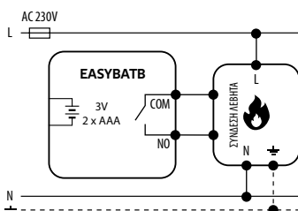
α) Διάγραμμα σύνδεσης στο λέβητα αερίου
