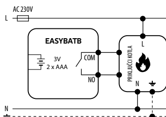
a) Šema povezivanja termostata sa gasnim kotlom
