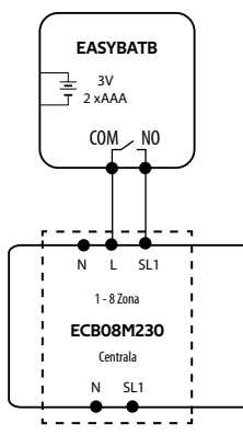
c) Šema povezivanja sa centralom
