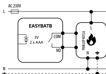
a) Vežalna shema za plinski kote
