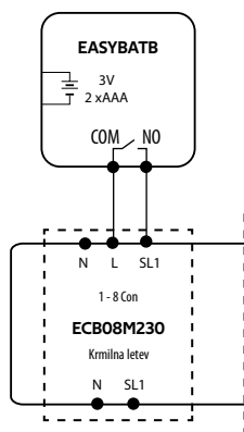
c) Vežalna shema za črpalke/pogon
