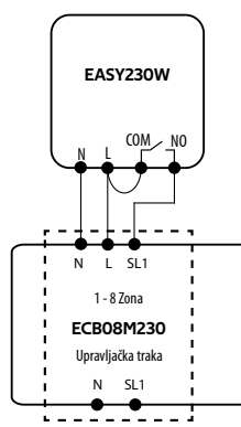
c) Shema spajanja na kontrolnu traku
