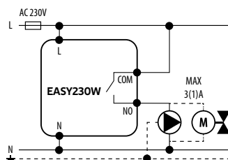
b) Shema priključka na pumpu / aktuator
