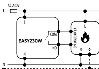
a) Shema priključka na plinski kotao
